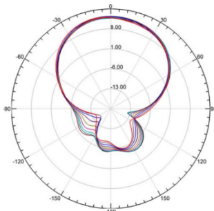
H-Pattern
