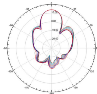
V-Pattern
