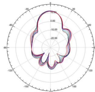
V-Pattern
